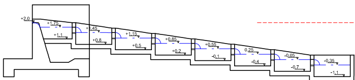
ΤΟΜΗ A-A
