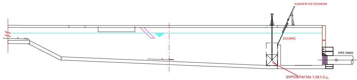
ΤΟΜΗ ΚΑΤΑ ΜΗΚΟΣ ΤΟΥ ΑΞΟΝΑ ΕΞΑΜΜΩΤΗ
